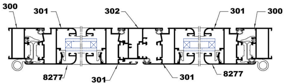
SECCION A-A
