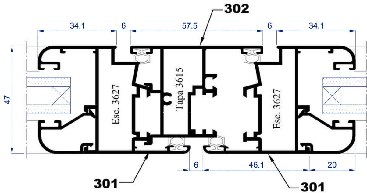
Nudo Central ventana
