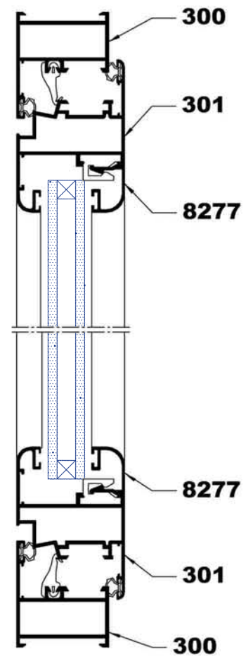
SECCION B-B
